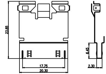
金屬下蓋
