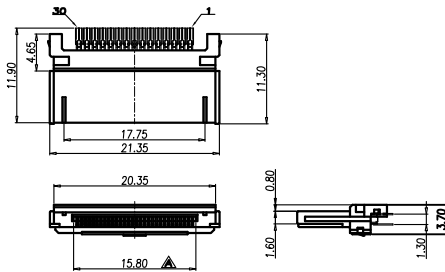
膠芯+PIN
