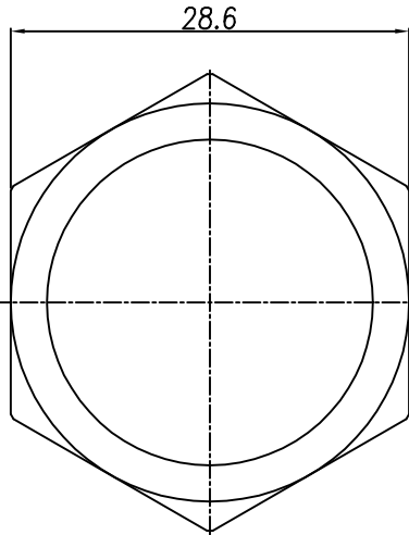
Hex Nut
