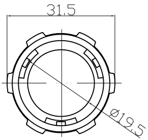
防水USB外螺母(黑色)
