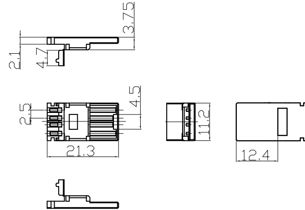
防水頭USB(M)膠芯+PIN
