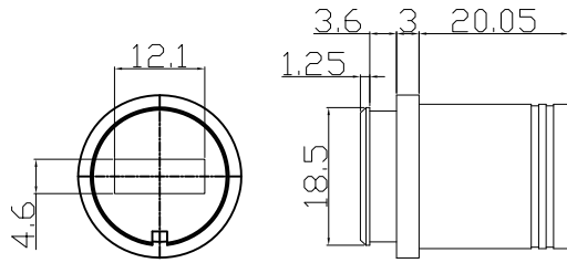
防水USB外螺母(黑色)
