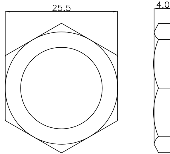
HEX NUT
