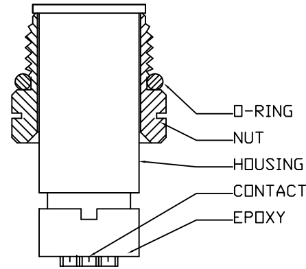
ASS'Y
